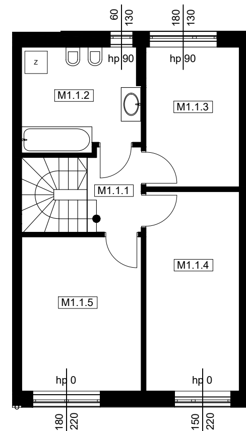
PIĘTRO
